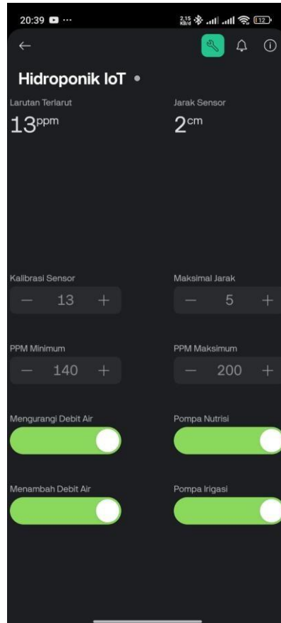
Gambar 6. Antarmuka Blynk
