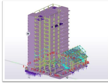
Gambar 2. Pemodelan Rencana Bangunan di aplikasi Tecla
