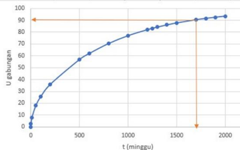
Grafik 1. Hubungan antara derajat konsolidasi (U) dan waktu (t) tanpa menggunakan PVD
