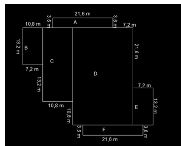
Gambar 4. Rencana Luas area rencana bangunan
